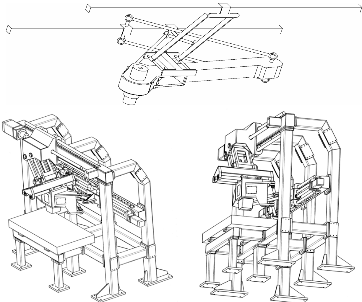
Slika 5. Dispozicija projektovanog prototipa mašine, pn101_4
