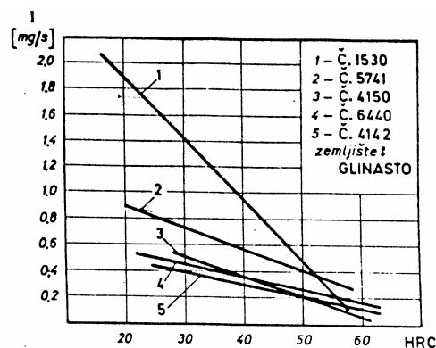
Sl. 8. Zavisnost istrošenja od tvrdoće materijala
