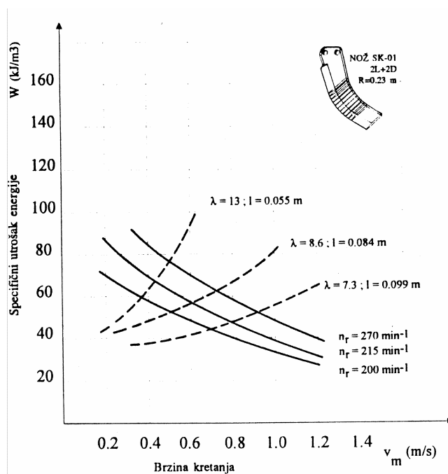
Sl. 4. Promena specifičnog utroška energije za obradu zemljišta sa rotacionim radnim elementima
