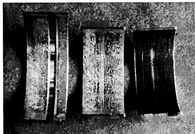
Slika 6 Površina ležaja oštećena abrazijom
