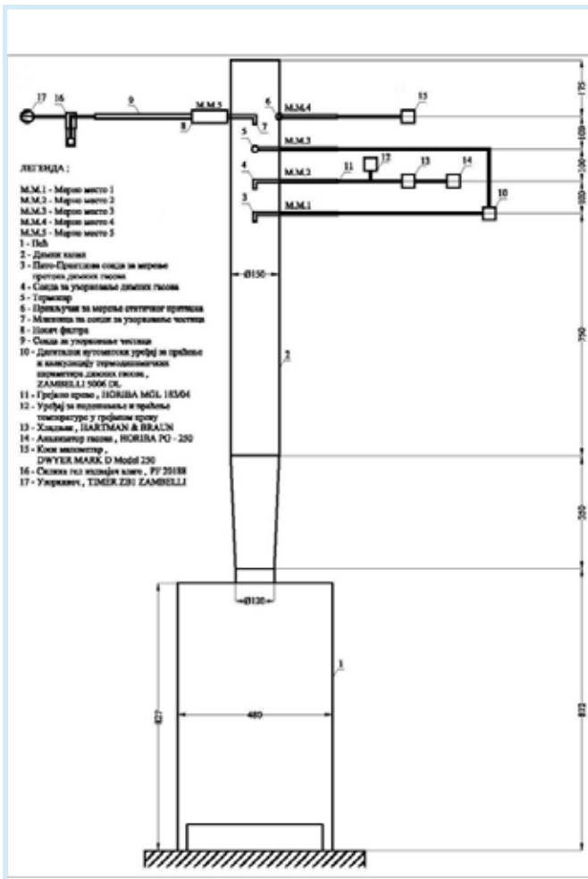
Slika 2. Šema eksperimentalne instalacije i mernih mesta
