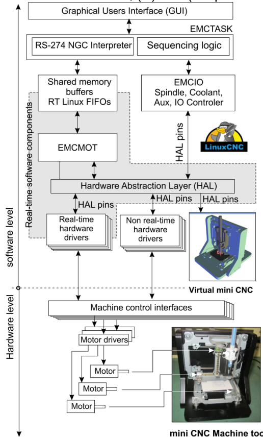
Fig. 7 ArchitectureLinuxCNC-afor mini CNC machine tool
