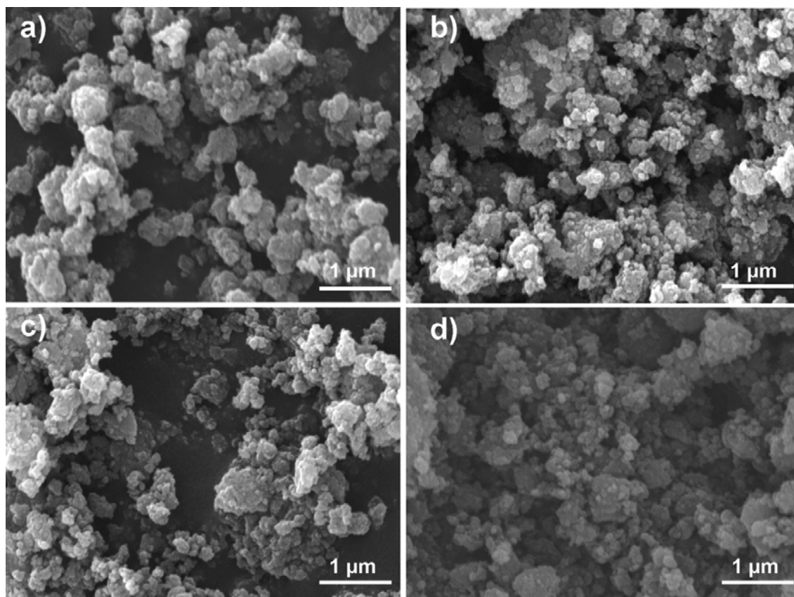
Figure 2. SEM micrographs of TiO 2 -0 (a), TiO 2 -10 (b), TiO 2 -30 (c) and TiO 2 -60 (d)
