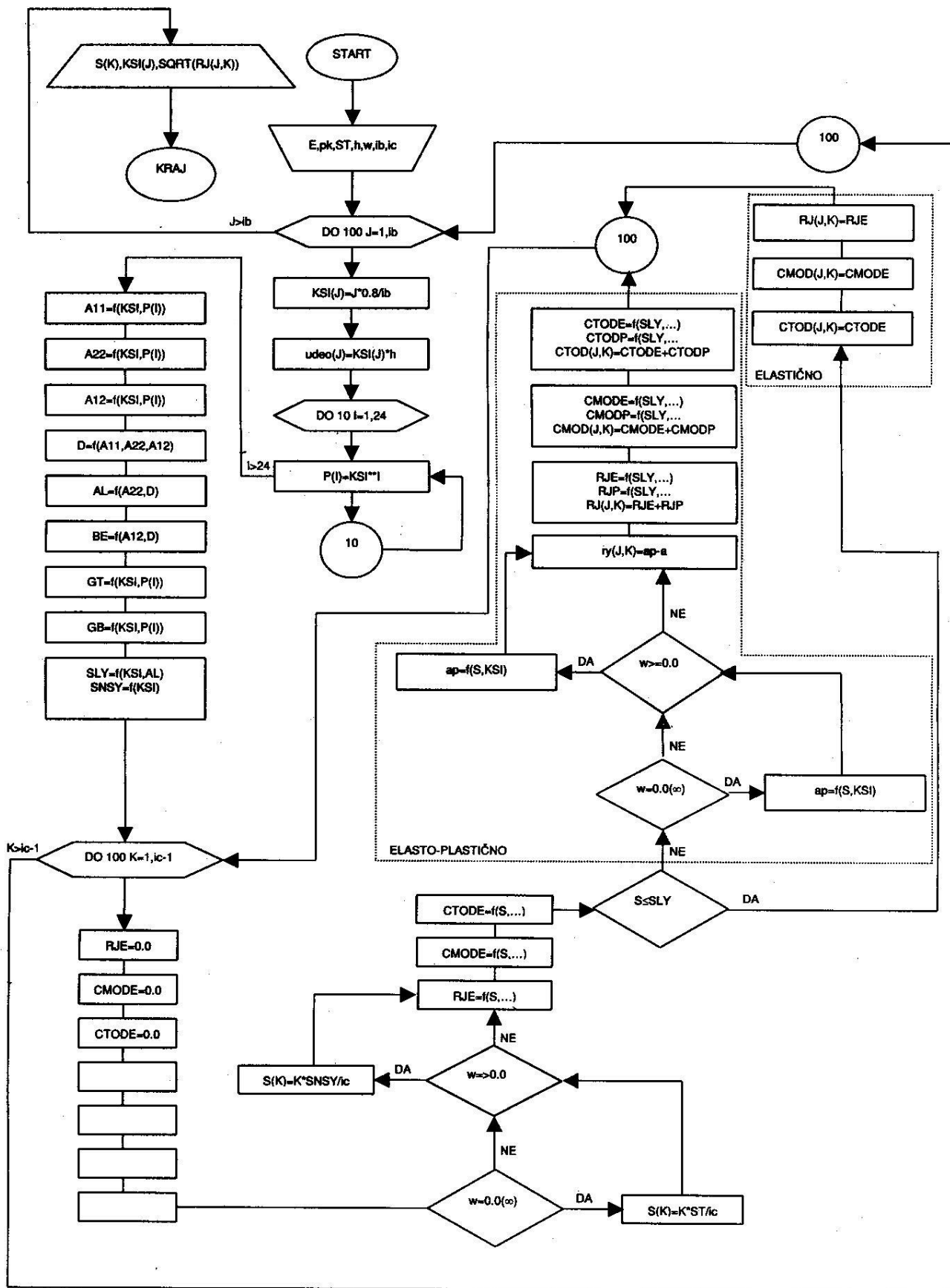
Slika 3. Algoritam za izradu programa KING0 i KING1 /5/
