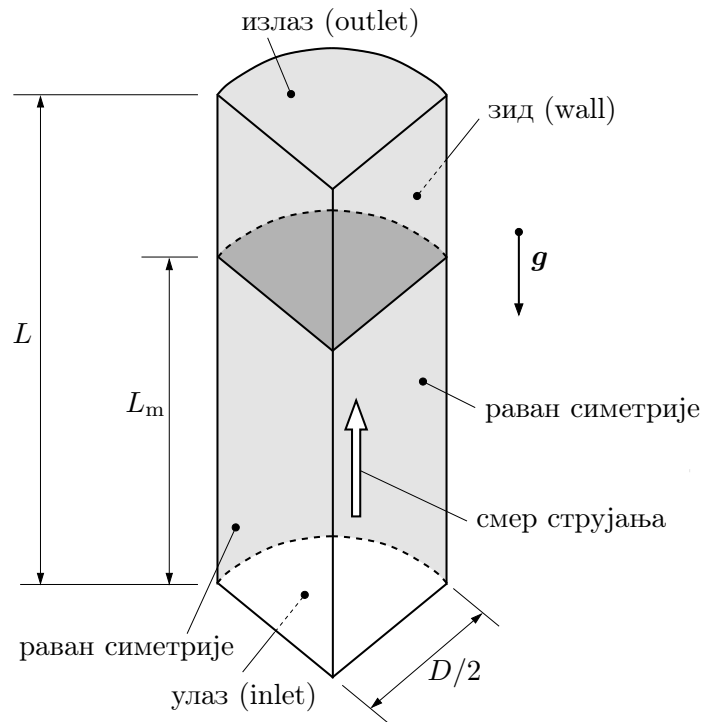
Слика 5.1. Прорачунски домен облика четвртине цеви.
