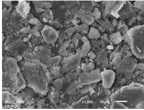
Slika 2. SEM mikrografija polaznog uzorka pirofilita.
