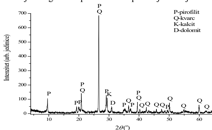
Slika 1. Difraktogram praha polaznog uzorka pirofilita.
